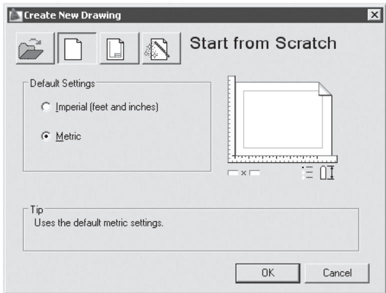
Рис. 1.3. Диалоговое окно создания нового рисунка
