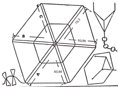
Рис. 4. Высотный змей № 1
