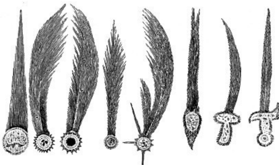
Старинные изображения комет.
