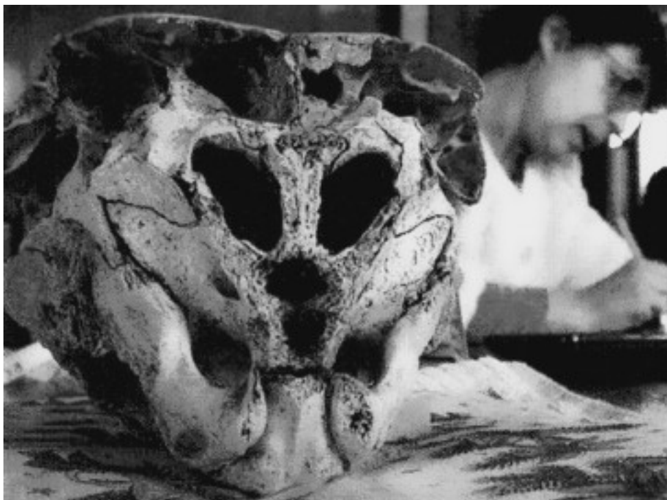
Череп болгарского циклопа, найденный в Родопских горах.
