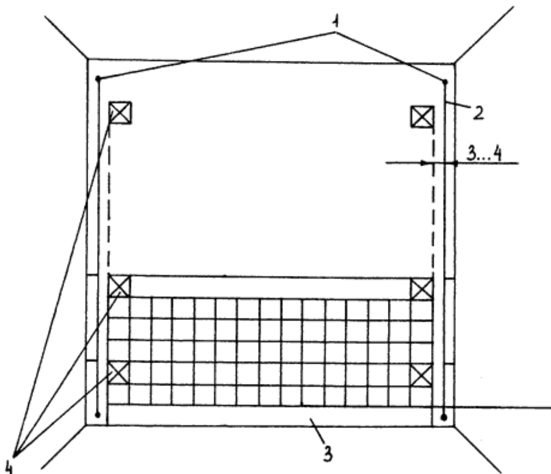
Рис. 8. Облицовка стен плиткой по маякам: 1 – гвозди; 2 – шнур отвеса; 3 – маячные плитки; 4 – причальный шнур
