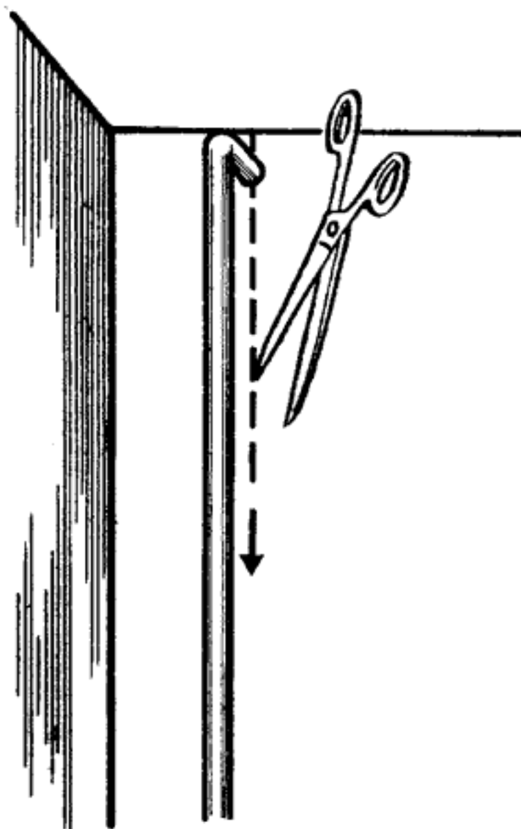
Рис. 6. Разрезание полотна, проходящего под трубой
