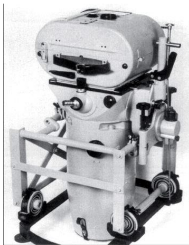
Широкоформатная автоматическая аэрофотокамера Rb 50/30 на раме, на которой она устанавливалась в фюзеляже самолета
