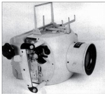
Ручная аэрофотокамера модели НК 19
