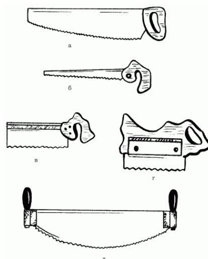
Рис. 16. Виды ножовок: а – поперечная широкая; б – узкая; в – с обушком; г – ножовка-наградка; д – двуручная поперечная пила.
