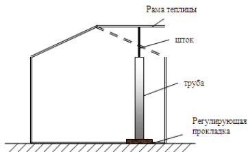
Рис. 2. Монтаж гидроцилиндра
