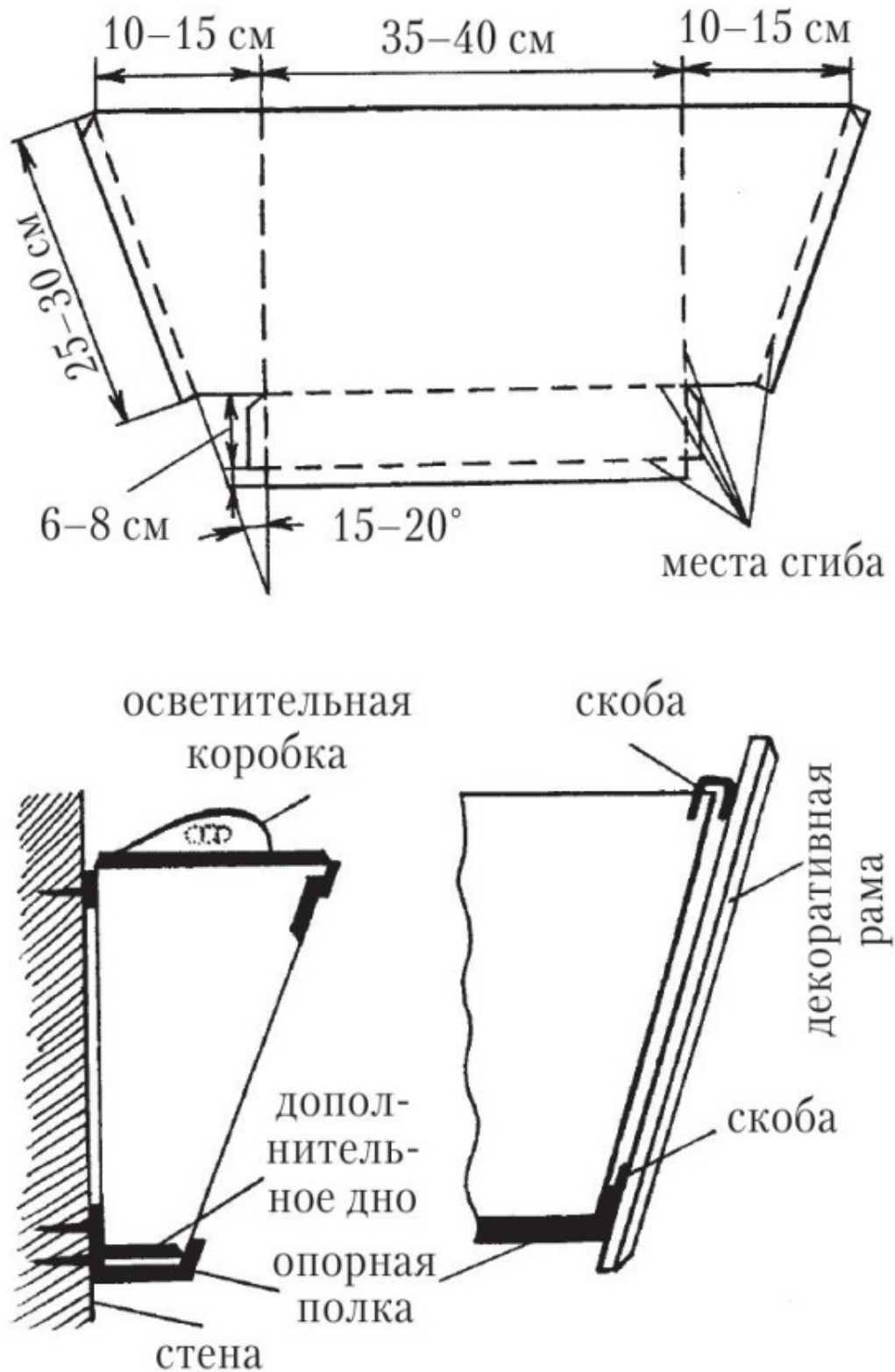
Рис. 4. Контуры развертки аквариума$картины
