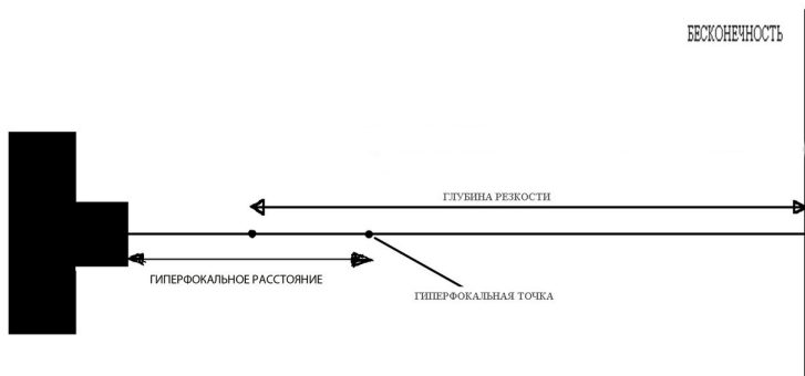
Рис 1. Глубина резко изображаемого пространства (ГРИП).
