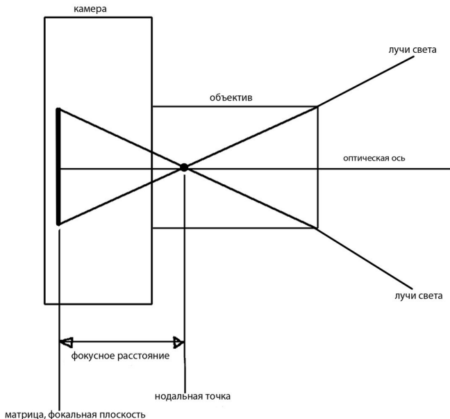
Рис 2. Фокусное расстояние и нодальная точка.
