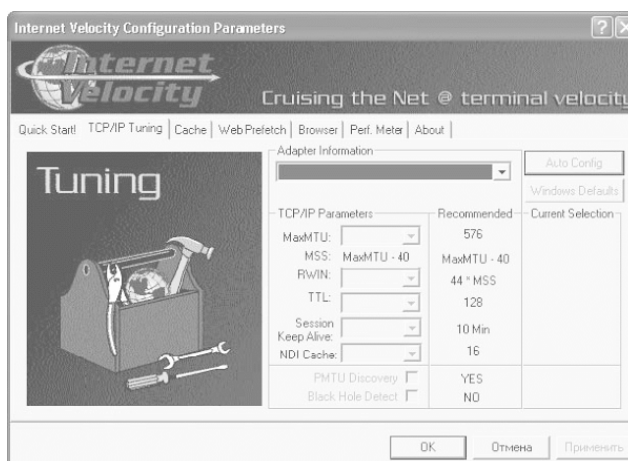
Рис. 1.6. Вкладка TCP/IP Tuning
