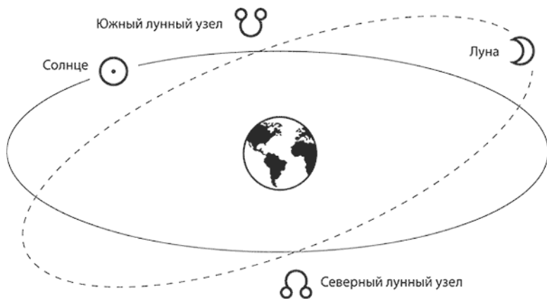
Рис. 27.1. Лунные узлы – пересечение путей Солнца и Луны
