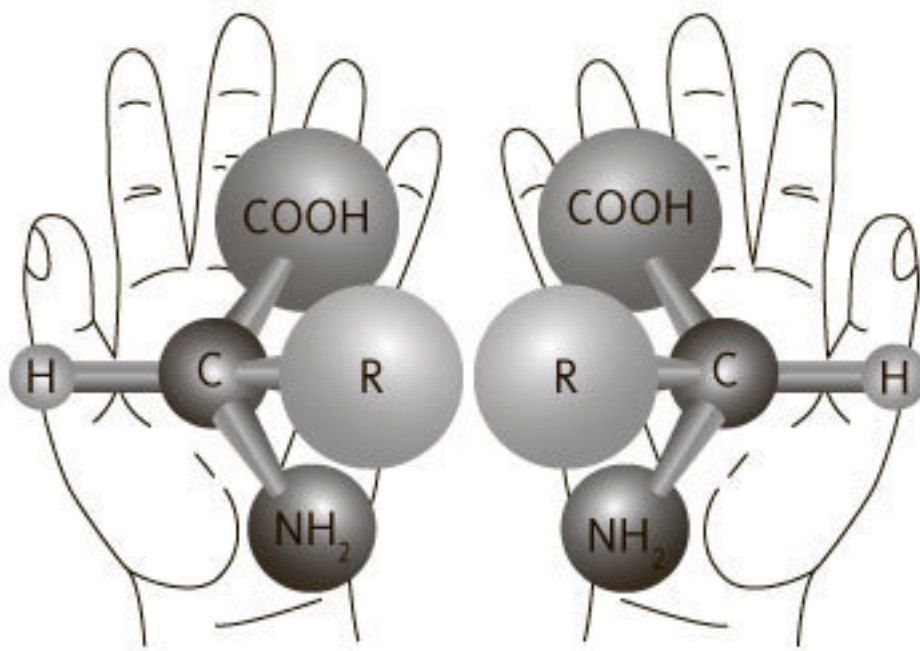
Рис. I.2. Молекулы-стереоизомеры
