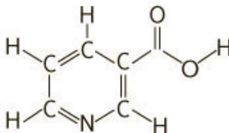
Рис. I.1. Молекулярное соединение
