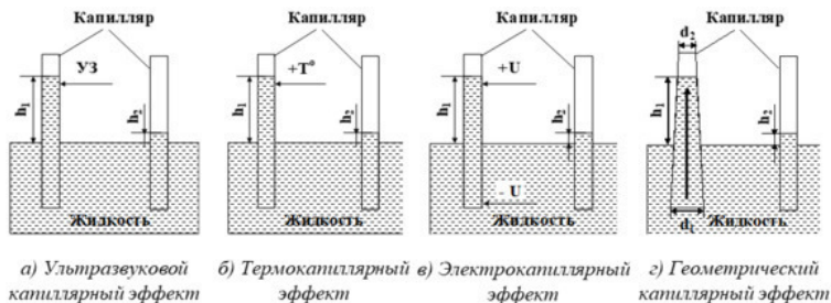
Рис. 5.52. Капиллярные эффекты
