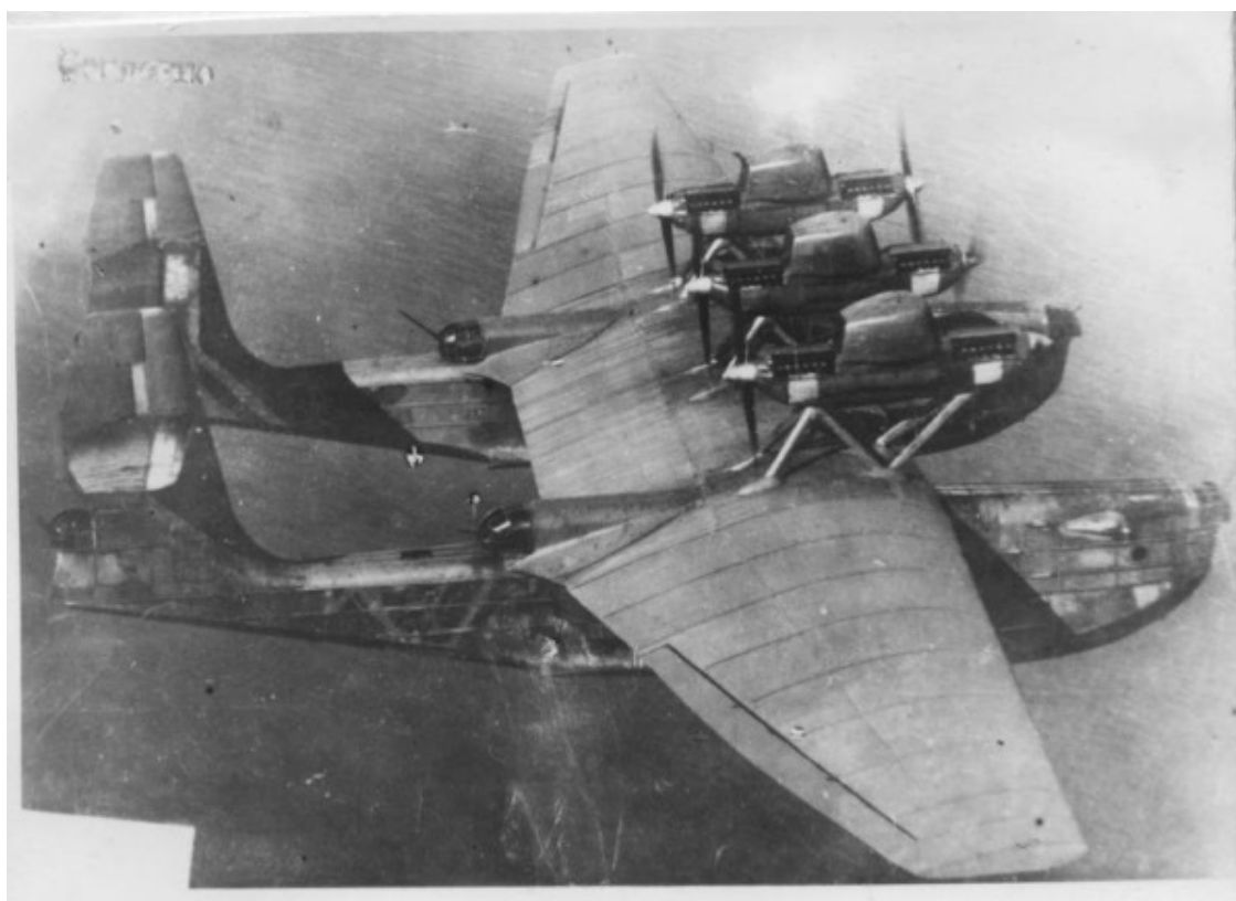
Гидросамолет АНТ-22 с закрепленными на фюзеляже аэро-подводными самодвижущимися снарядами (АПСС)
