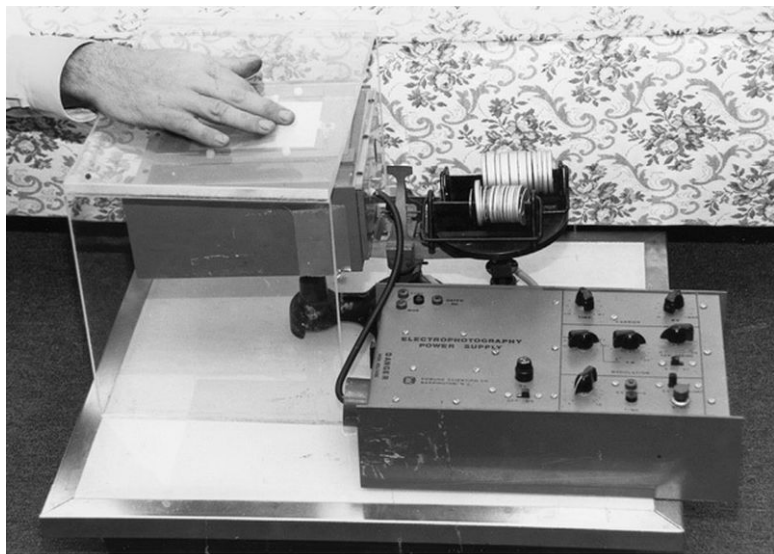
Рис. 1. Экспериментальная установка для получения электрофотографических изображений
