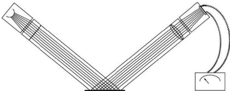
Рис. 6. Теоретическая модель количественной оценки кирлиановой электрофотографии
