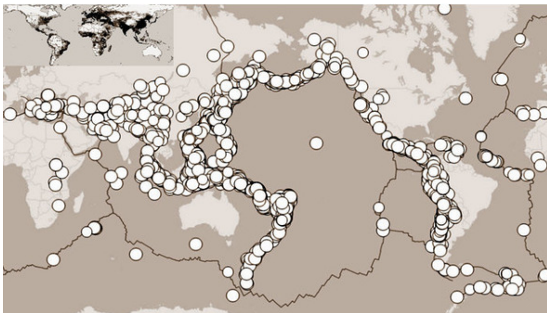
Расположение очагов сильнейших землетрясений магнитуды 7 и выше с 1900 по 2015 год. На верхней врезке карта плотности населения на планете (тёмные цвета).
