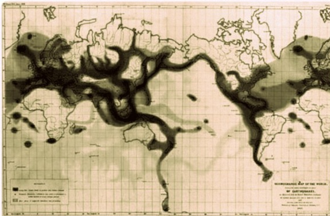
Карта мировой сейсмичности Роберта Маллета, 1854 год.
