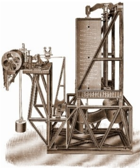
Сейсмограф Вихерта для записи сейсмических колебаний (из архива автора).
