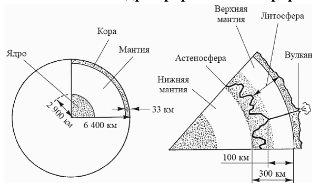
Рис. 4. Структура недр планеты (со схематическим вулканом)
