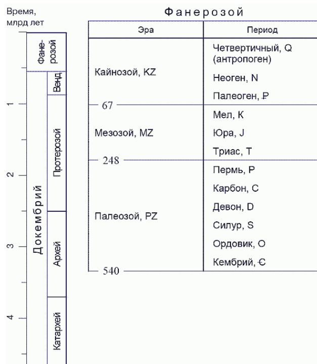
Рис. 2. Геохронологическая шкала. Для того чтобы запомнить последовательность периодов, составляющих фанерозой (кембрий, ордовик, силур, девон, карбон, пермь, триас, юра, мел, палеоген, неоген, антропоген), студенты испокон веков пользуются мнемонической фразой не вполне педагогического свойства: «Каждый отдельный студент должен купить пол-литра. Ты, Юрик, мал – подожди немного, а то...»
