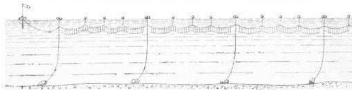
Рис. 4. Английская белужья снасть
