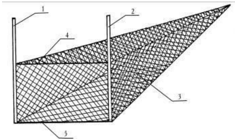
Рис. 11. «Курица»: 1,2 – клячи; 3 – мотня; 4 – верхний шнур; 5 – нижний шнур.
