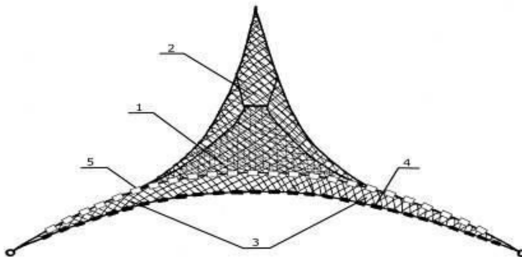
Рис. 13. Положение бредня-ловушки при ловле (вид сверху): 1 – мотня-горло; 2 – мотня-кутец, 3 – крылья; 4 – грузовой шнур; 5 – наплавной шнур.
