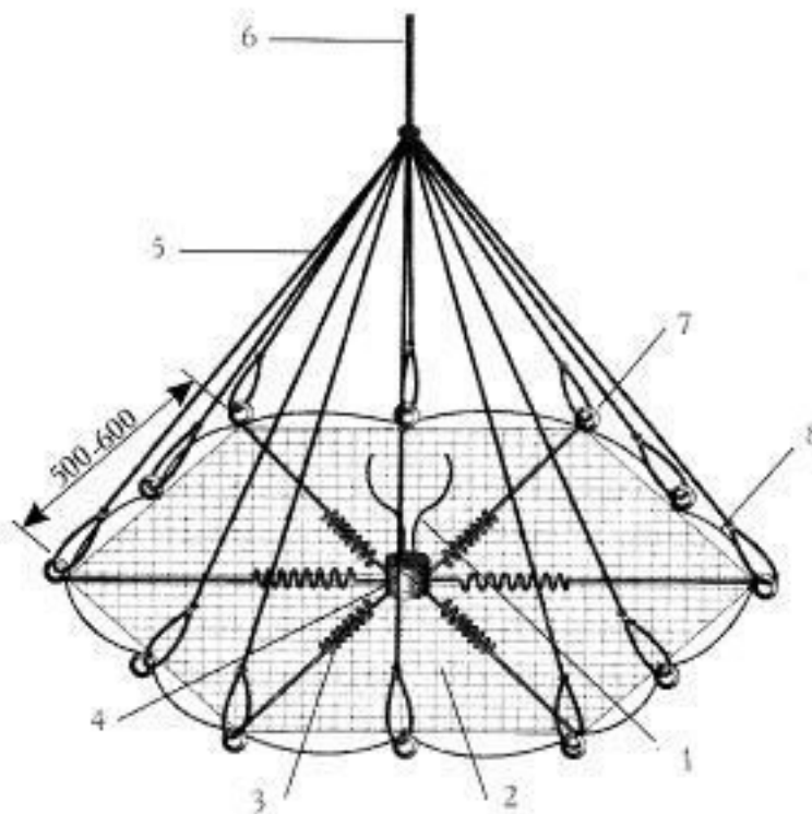
Рис. 16. Подъемник-«зонтик» конструкции Д. Звягинцева: 1 – проволочки для привязывания приманки; 2 – сетное мелкоячеистое полотно; 3 – пружинные распорки; 4 – свинцовый груз весом 100 г; 5 – стропы; 6 – тяговый шнур, 7 – кольца, 8 – боковая нить.
