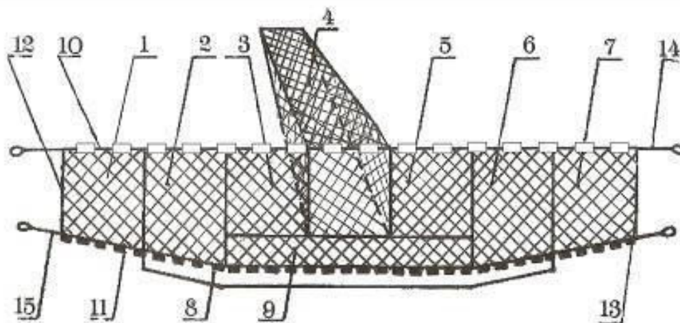
Рис. 8. Бредень и его составные части: 1 – правое крыло (2 часть); 2 – правое крыло (1 часть), 3 – правый привод; 4 – мотня; 5 – левый привод; 6 – левое крыло (2 часть); 7 – левое крыло (1 часть); 8 – подзор; 9 – сорочка; 10 – верхняя подбора; 12 – правый кляч; 13 – левый кляч; 14 – верхняя чалка; 15 – нижняя чалка.
