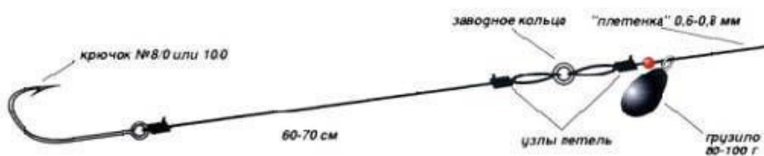
Рис. 5. Оснастка белужьей снасти (по О. Соболеву)
