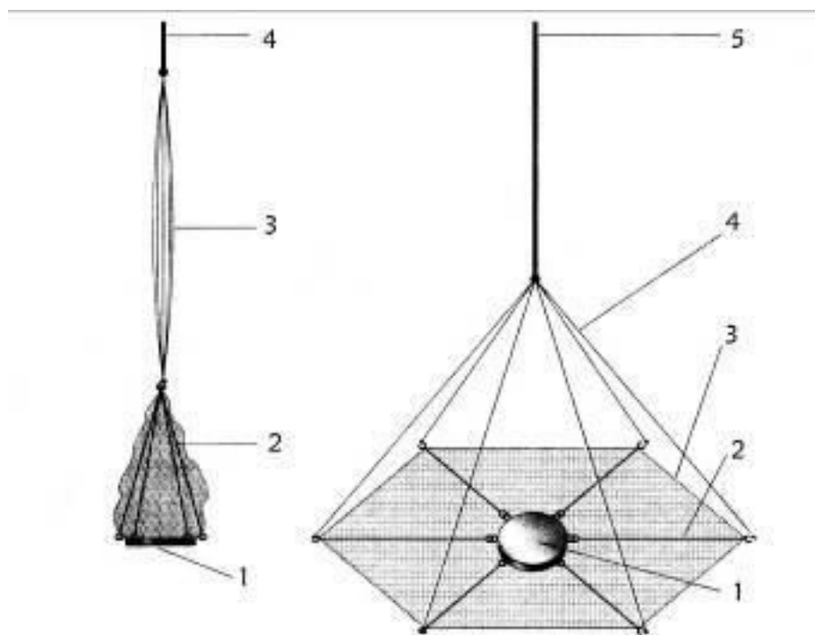
Рис. 15 Подъемник-«зонтик» конструкции В. Золотарева: 1 – медная шайба диаметром 40 мм; 2 – спицы длиной 480 мм из проволоки диаметром 5 мм, подвижно соединенные с шайбой; 3 – леска, соединяющая концы спиц; 4 – стропы; 5 – тяговый шнур.
