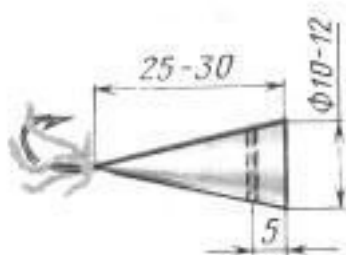
Рис. 7. Мормышка «конус» с крючком, замаскированным красной шерстью.
