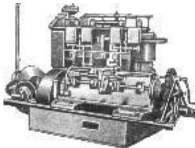
Двигатель управляемого аэростата Шварца
