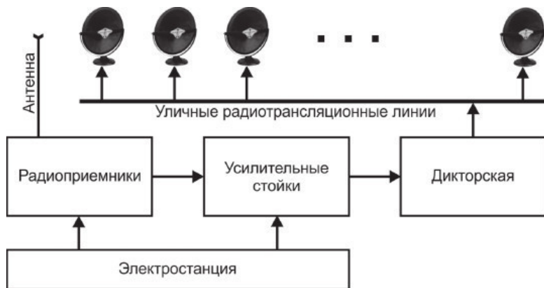
Схема районного радиоузла
