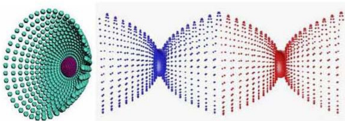
Фото 2.2. Схема волновода фотона из зёрен-электропотенциалов
