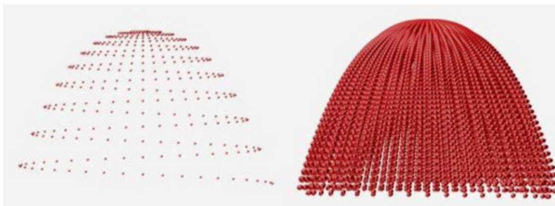
Фото 2.6. Лёгкие атомные и «тяжёлые» СВЧ – фотоны
