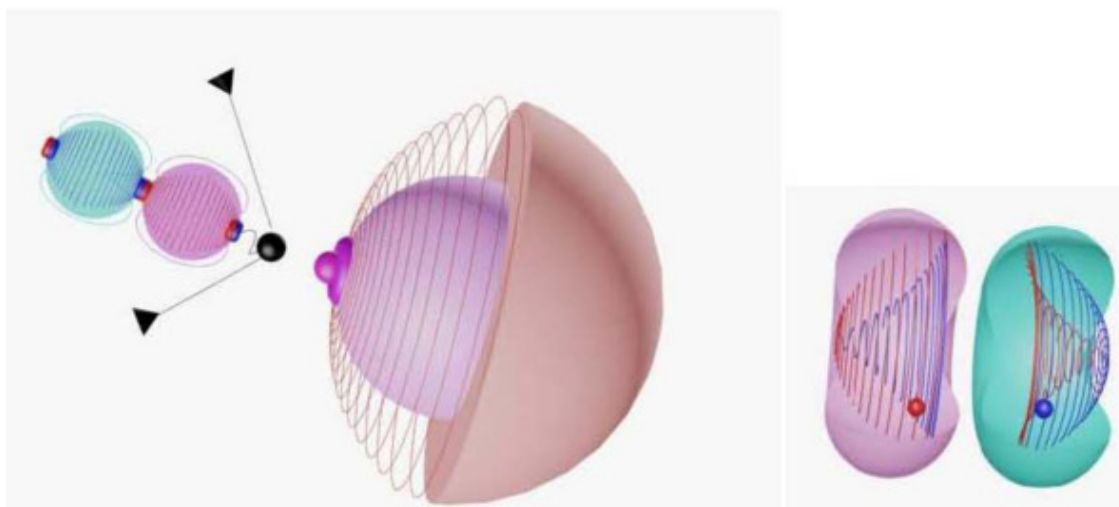
Фото 2.5. Схема рождения пары в поле атомного ядра
