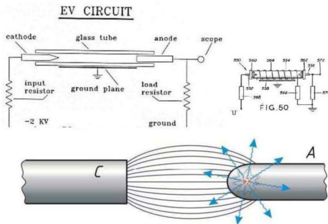
Фото 2.13. Реактор зарядовых кластеров К. Шоулдерса (вверху) и реактор С. В. Адаменко (внизу)
