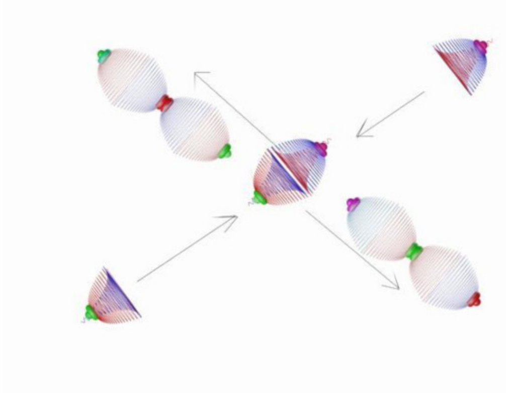
Фото 2.20. Аннигиляция пары электрон-позитрон
