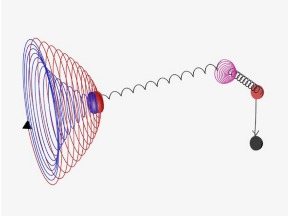
Фото 2.22. Схема распада мюона
