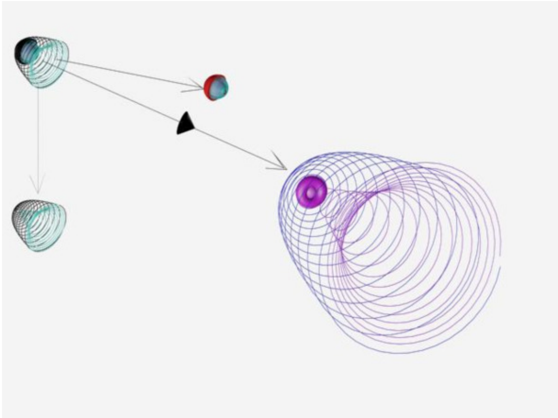
Фото 2.17. Распад нейтрона
