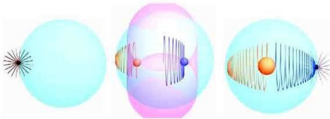
Фото 2.9. Изменения магнитного поля в фазовом объёме полволны
