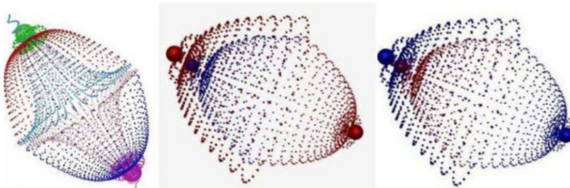
Фото 2.27. Схемы \pi – мезонов и структуры их волноводов
