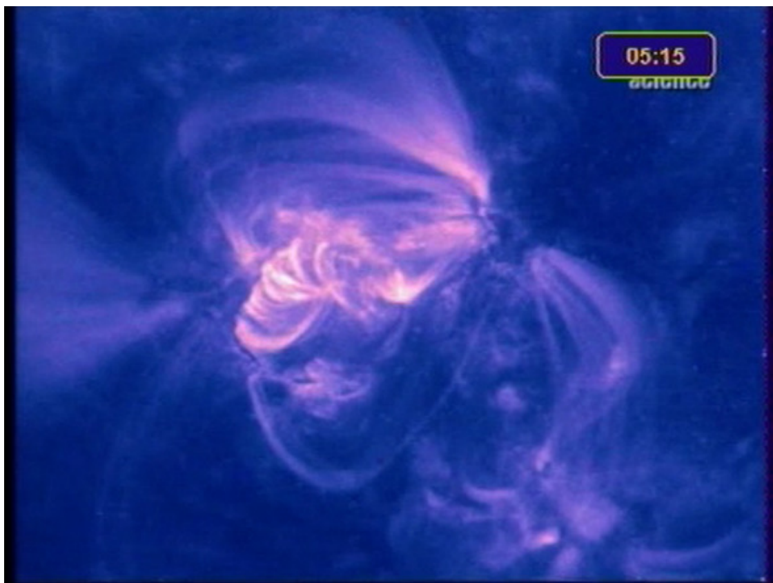
Фото 2.10. Магнитный диполь в хромосфере
