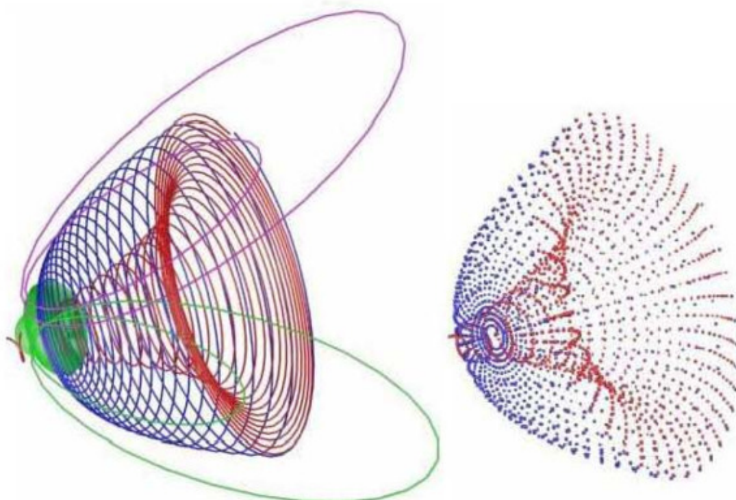
Фото 2.15. Схема электрона, обозначенная электро (синими) и гравпотенциалами (красными) его волновода ГЭММ и структура отбрасываемого контура из зёрен-потенциалов, который формирует его внешнее поле.
