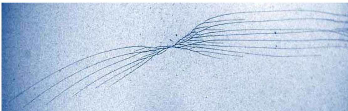
Фото 2.14. Треки гиперзвука из точки поглощения кванта ВЧ-излучения с рождением ГЭМД, излучающего гиперзвук.
