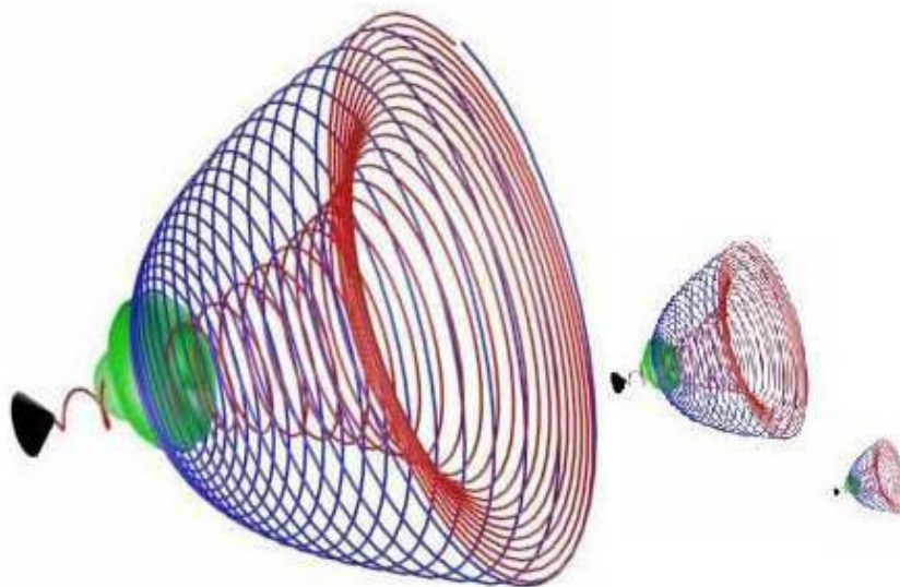
Фиг. 2.23 Сравнение схемы и размера четверть-волноводов электрона (слева), мюона (посредине) и тау-лептона (справа).
