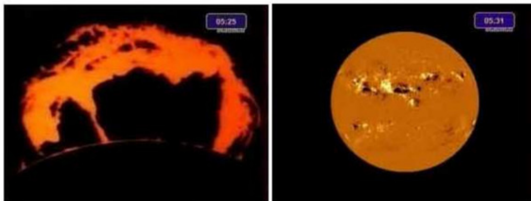
Фото 2.7. Кластер фотосферы, захваченный гигантским гипермонополем и Пары «чёрных и белых» пятен (справа).
