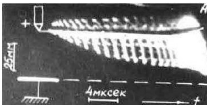
Фото 2.3. Картина электроразряда в жидкости
