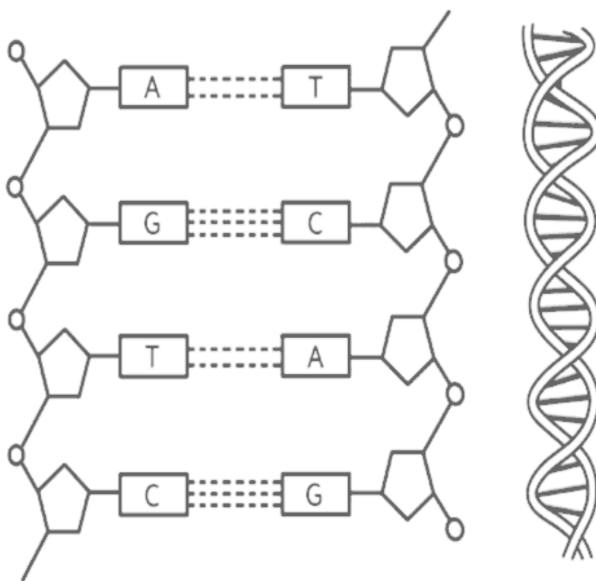
Строение ДНК
