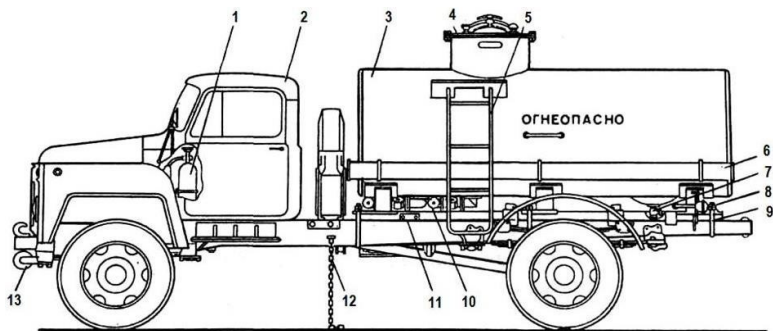
Рисунок 1 – Автомобиль-цистерна АЦ-4,2-53А:
