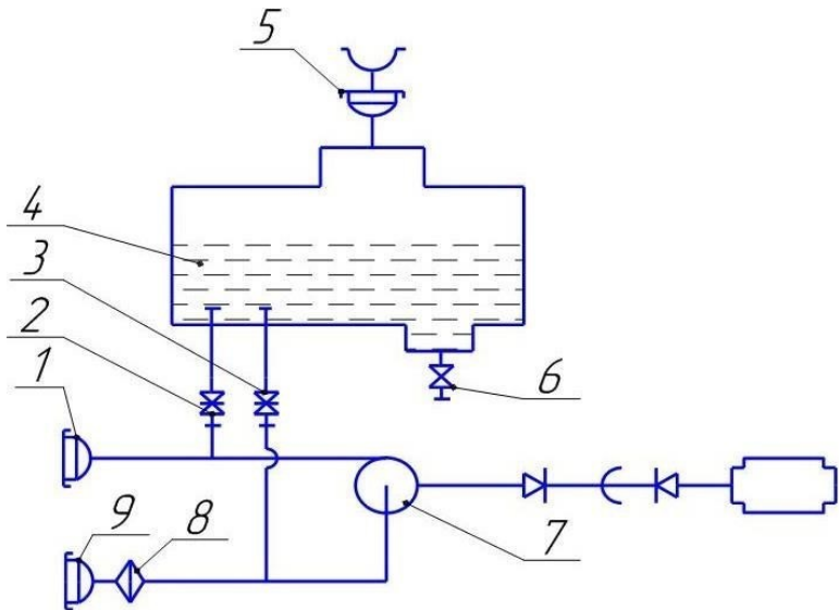
Рисунок 2 – Технологическая схема автомобиля-цистерны АЦ -4.2-53А:
