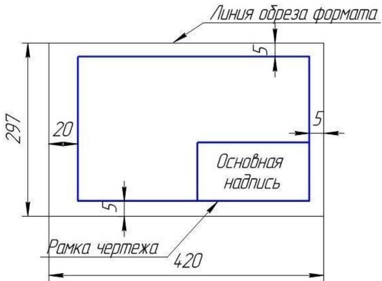
Рисунок 1 – Выделение формата А3 и выполнение рамки чертежа
