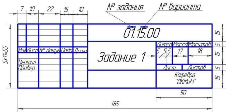
Рисунок 2 – Размеры и пример заполнения основной надписи
