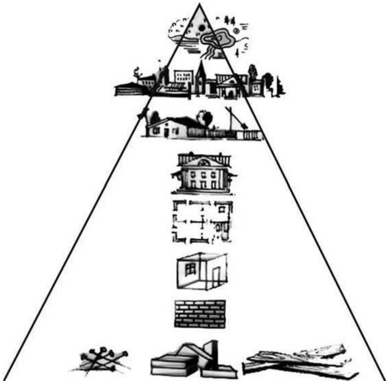
Рис. 3.1. Территориальная система (строительные материалы → населенные пункты)
