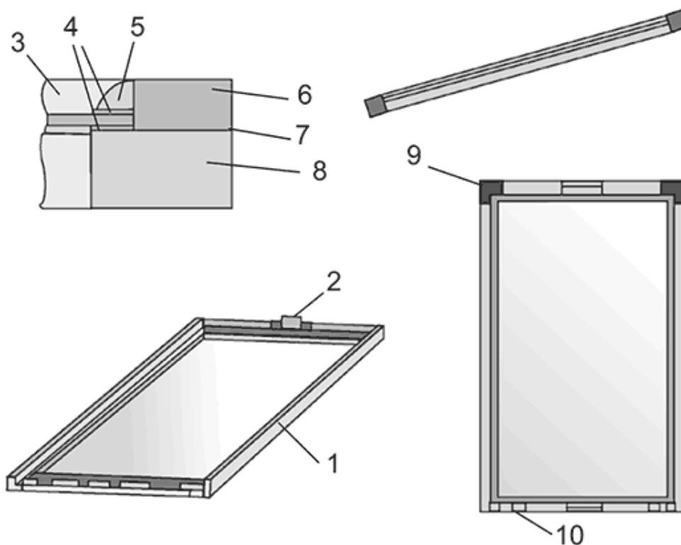
Рис. 8. Изготовление парниковых рам: 1 – рама по размеру стекла; 2 – ручка; 3 – стекло; 4 – замазка с двух сторон; 5 – штапик или гвозди с замазкой; 6 – брусок 40 × 20 мм; 7 – место склейки водостойчивым клеем; 8 – брусок 55 × 30 мм; 9 – стальной угольник; 10 – накладка для упора.
