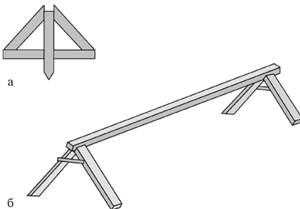
Рис. 3. Двускатные укрытия.
