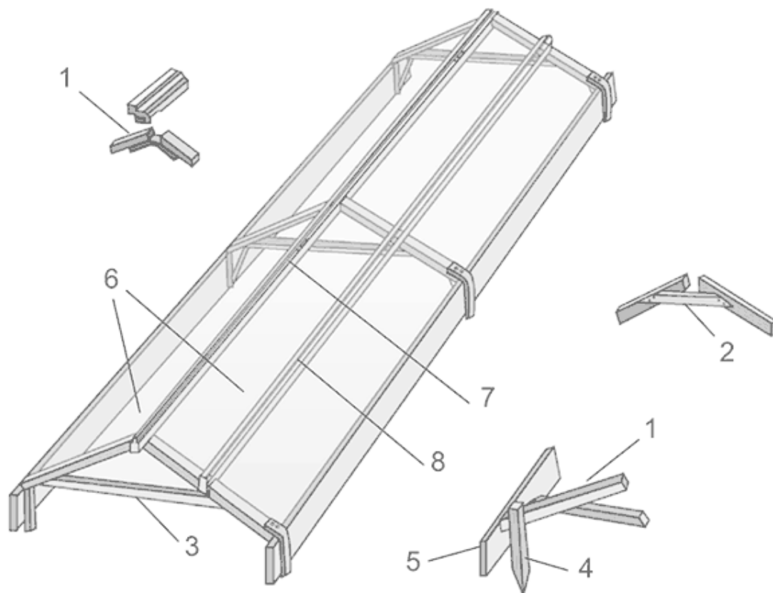
Рис. 4. Укрытие разборно-приставное: 1 – стропильный брус; 2 – накладка; 3 – стяжка; 4 – колышек; 5 – бортовая доска; 6 – пленочное покрытие; 7 – коньковый брус; 8 – бобина.
