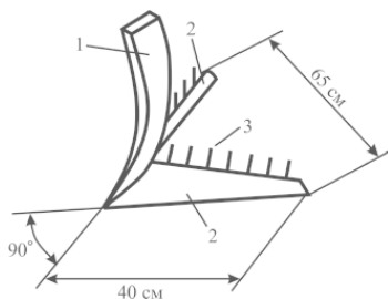
Рис. 5. Безотвальный рыхлитель
