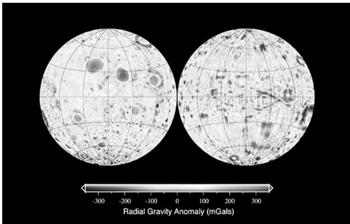
Карта гравитационных аномалий Луны. NASA
