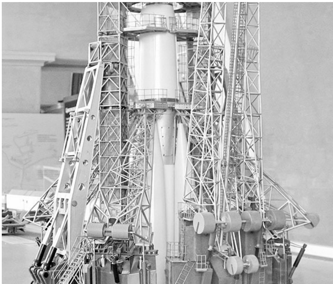
Часть макета стартовой площадки космодрома Байконур с системой «Тюльпан»
