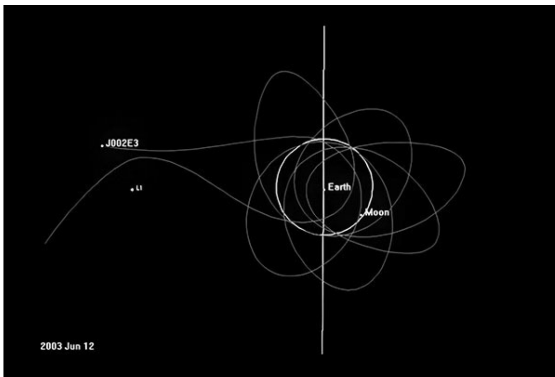
Орбита J002E3. NASA
