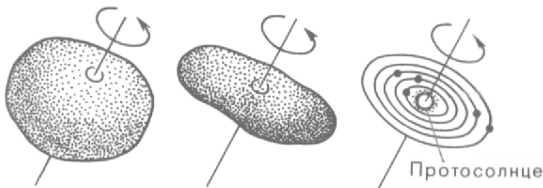
Рис.1. Эволюция протопланетного облака (схема)
