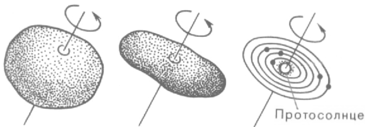
Рис.1. Эволюция протопланетного облака (схема)
