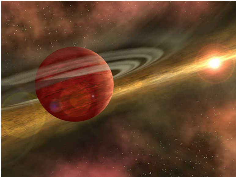
Рис.2. Молодая планета в протопланетном облаке
