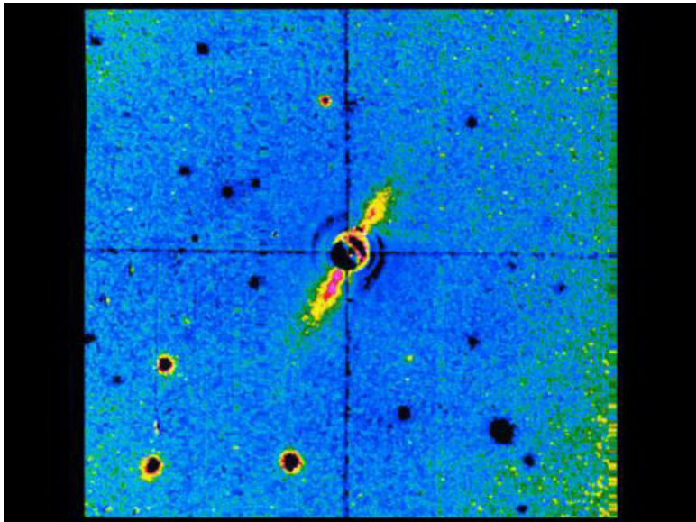
Рис.7. Бета Живописца (снимок с Земли)
