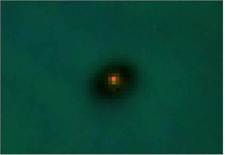
Рис.5. Протопланетный диск в Туманности Ориона
