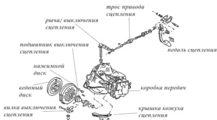
Рис. 3. Система сцепления в «Опеле Вектра»
