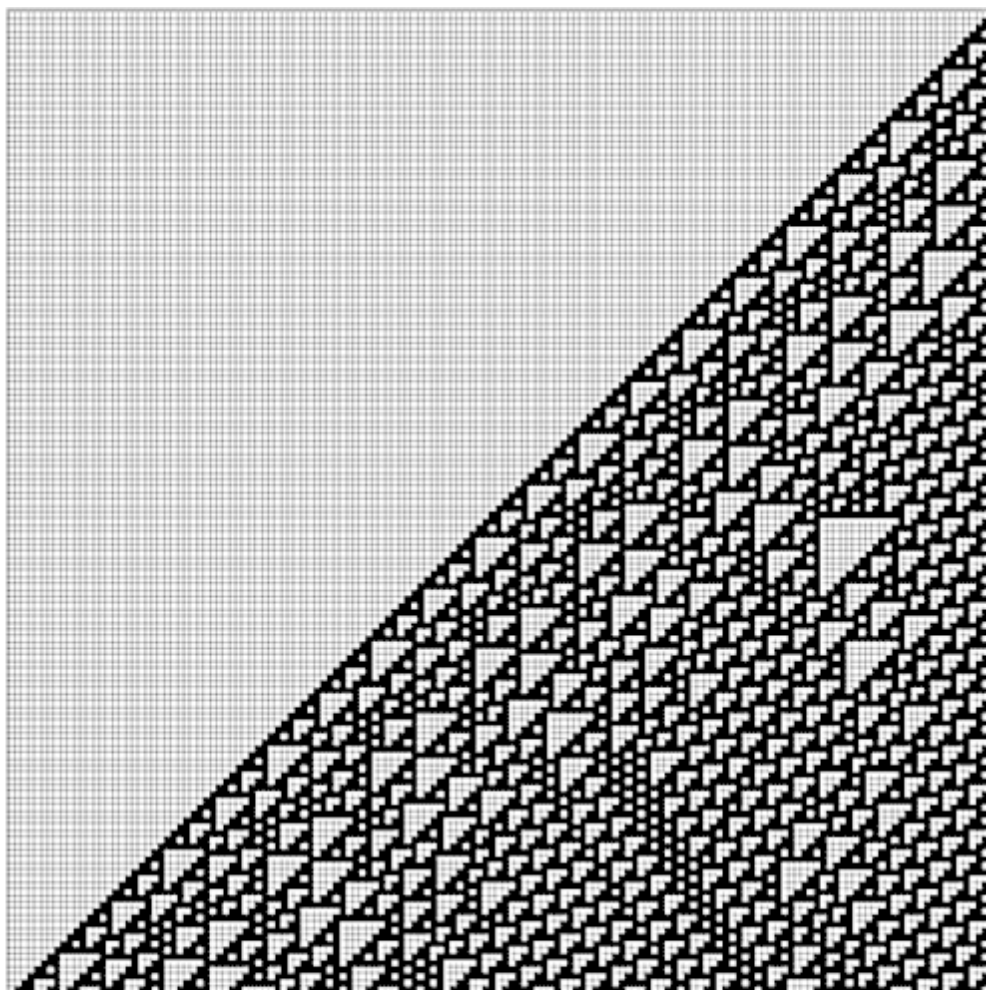
Илл 5.2. Клеточный автомат Стивена Вольфрама
