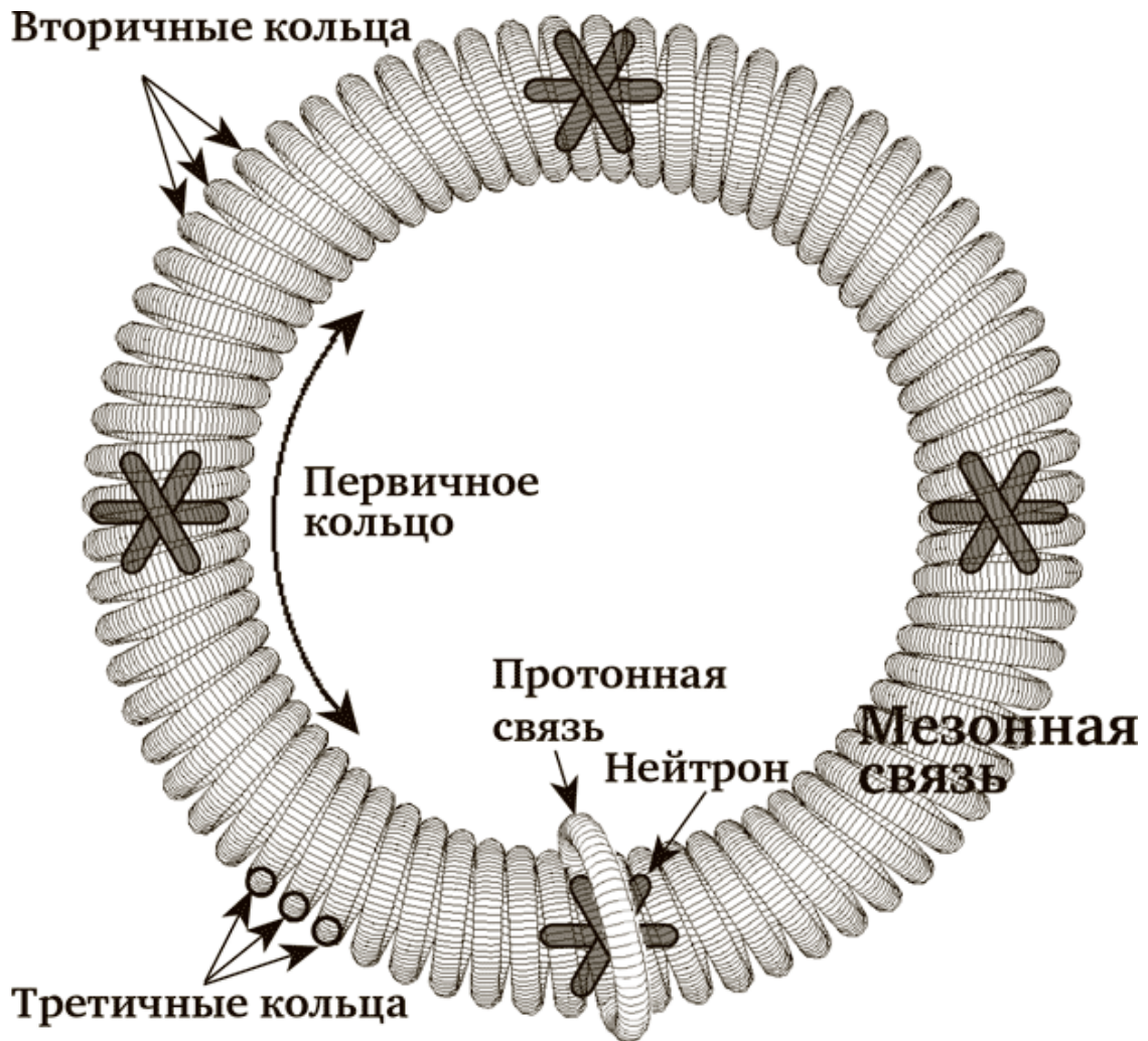
Илл. 5.1. Цирклоновая модель структуры ядра
