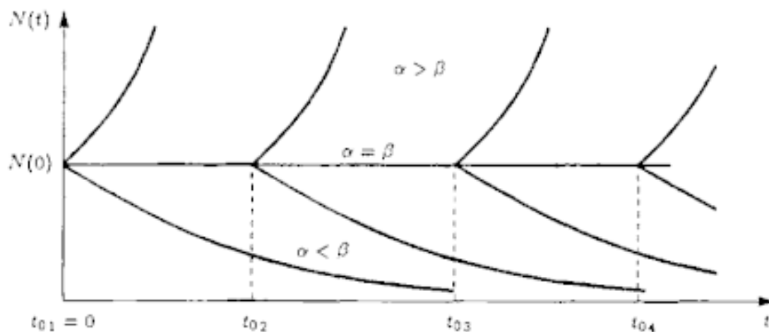
Изменение численности популяции со временем в модели Мальтуса ( \alpha – рождаемость; \beta – смертность)
